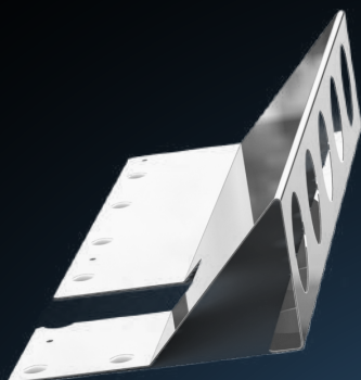
KW TOL01 A (PAR) TOLVA BASE PARA ESPEJO OREJON PARA KW 5 HOYOS PARA PLAFÓN 2" 1/4 T-660
