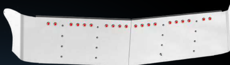
KW VC07 EE (KIT) VISERA KW T-680 / T-880 MOD B 20 HOYOS PARA PLAFÓN DE 3/4"
